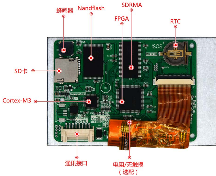
图 1-3 硬件配置图
