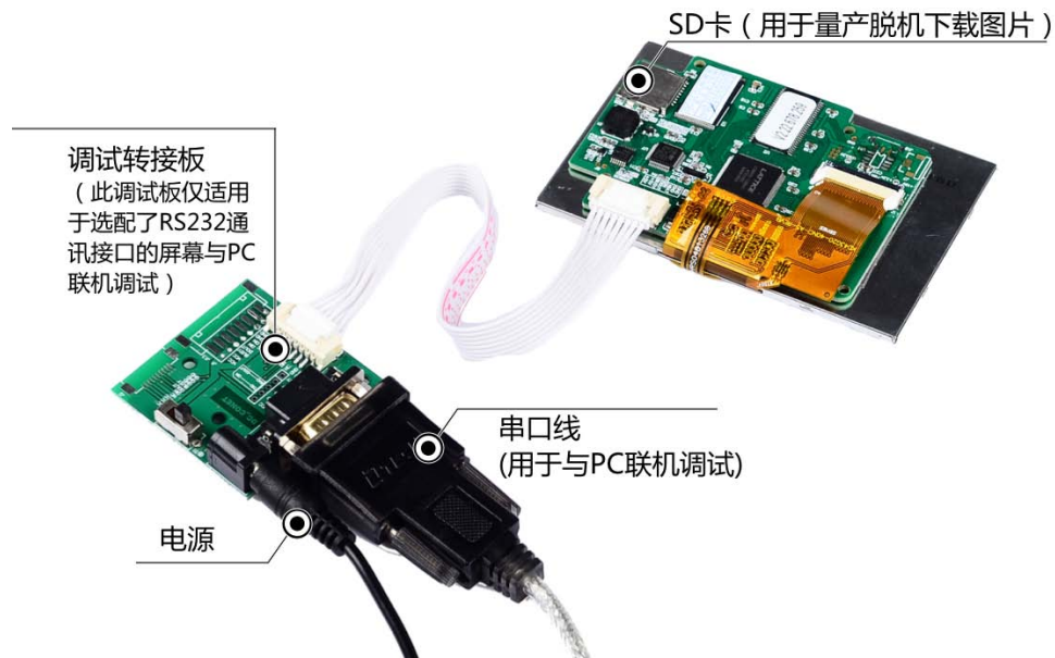
图 1-4 调试工具图
